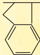
(Indene)
