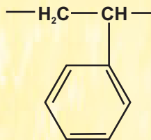
(Styrene)
